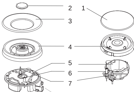
Конфорки с тройным рядом пламени
