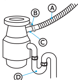
(A) Tuyau de vidange (B) Vis-Type de pince (C) Orifice d'admission des déchets (D) Siphon
