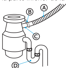
(A) Manguera de desagüe (B) Abrazadera de tornillo (C) Entrada del triturador de basura (D) Trampa de drenaje
