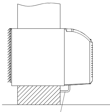
CHEMINEMENT DU CÂBLE DU THERMOSTAT (SOUS LE MANCHON, DERRIÈRE LE PANNEAU AVANT)
