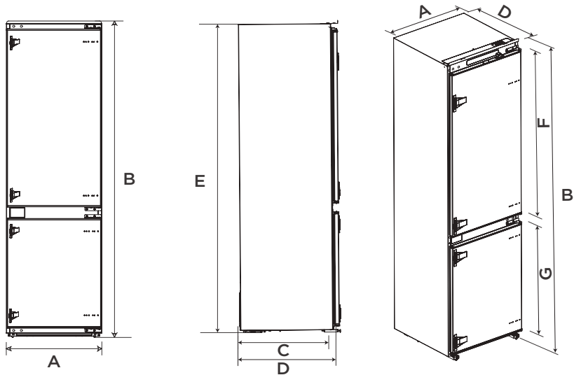
Diagrama do espaço necessário (com a porta aberta e com a porta fechada)
