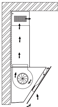
Recirculation mode
