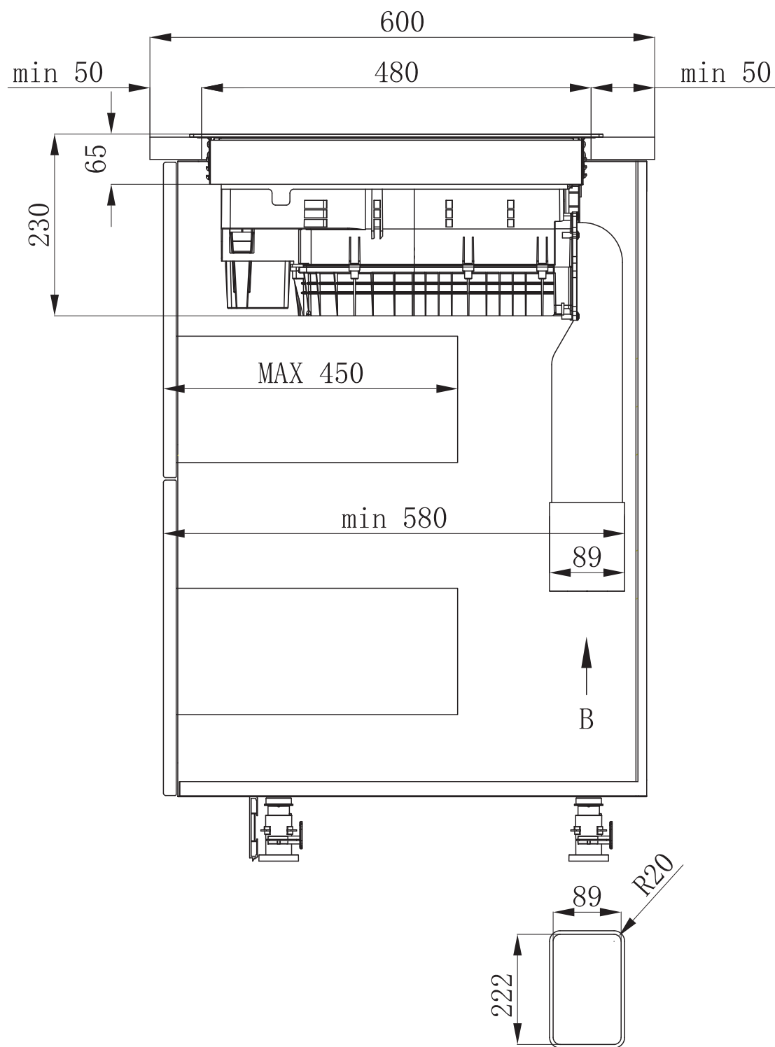
Vue : Dimension de l'adaptateur
