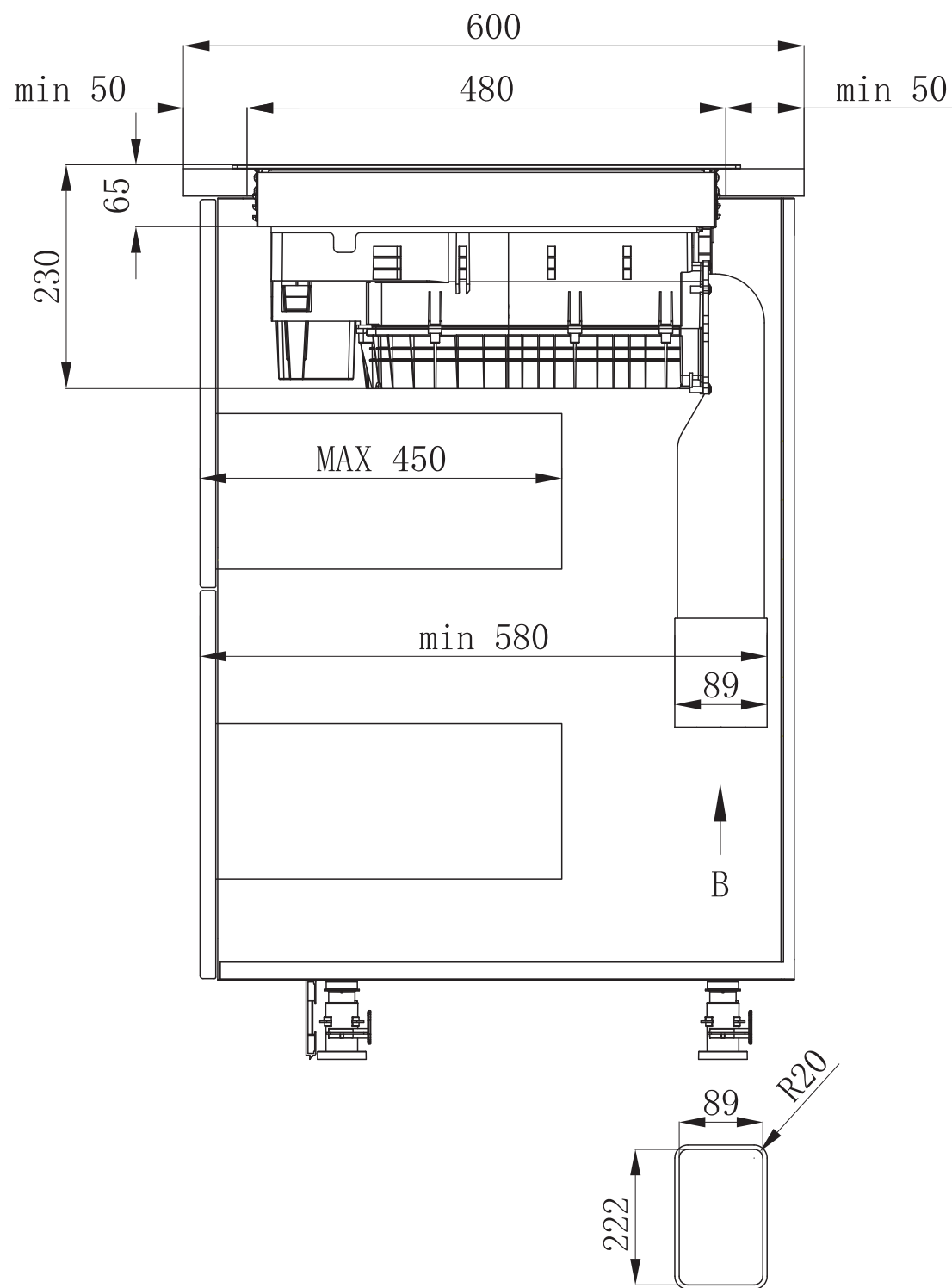
Vista: Dimensioni dell'adattatore
