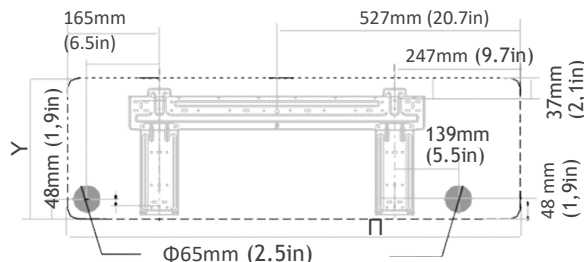
Διαστάσεις εσωτερικής μονάδας (Πλάτος x Ύψος): 971mm(31,7in)x321mm(11,6in)
