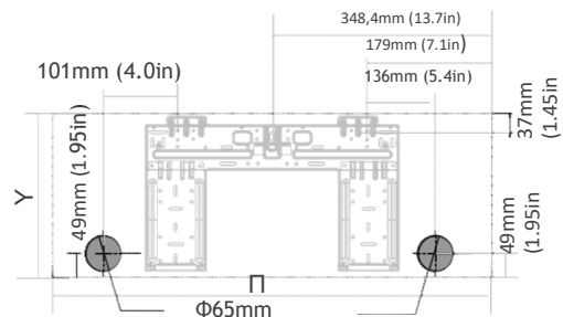
Διαστάσεις εσωτερικής μονάδας (Πλάτος x Ύψος): 729mm(28,7in)x292mm(11,5in)
