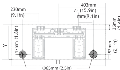
Διαστάσεις εσωτερικής μονάδας (Πλάτος x Ύψος): 805mm(31,7in)x295mm(11,6in)
