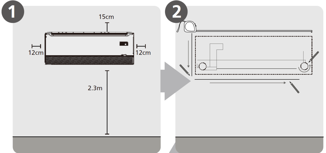
Definizione della posizione sulla parete
