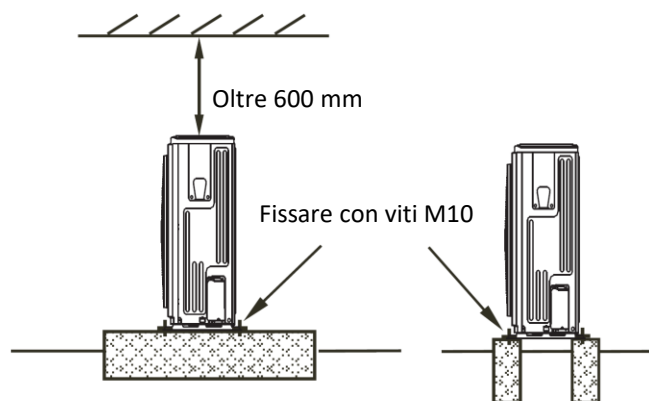
Schema Dimensionale
