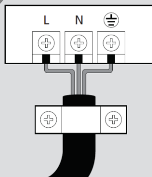
Cablaggio elettrico
