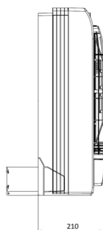
Vista laterale
