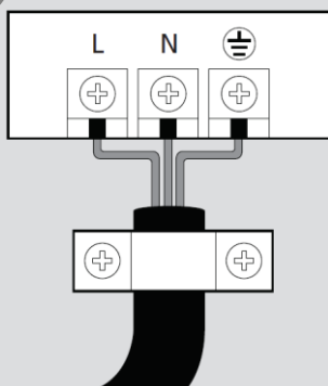
Cablaggio elettrico
