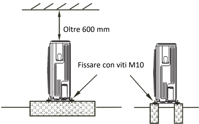
Schema Dimensionale
