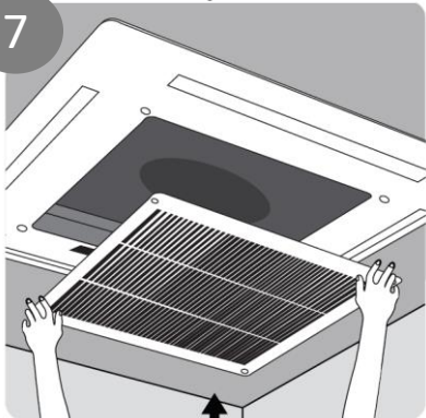
Installazione Pannello Decorativo
