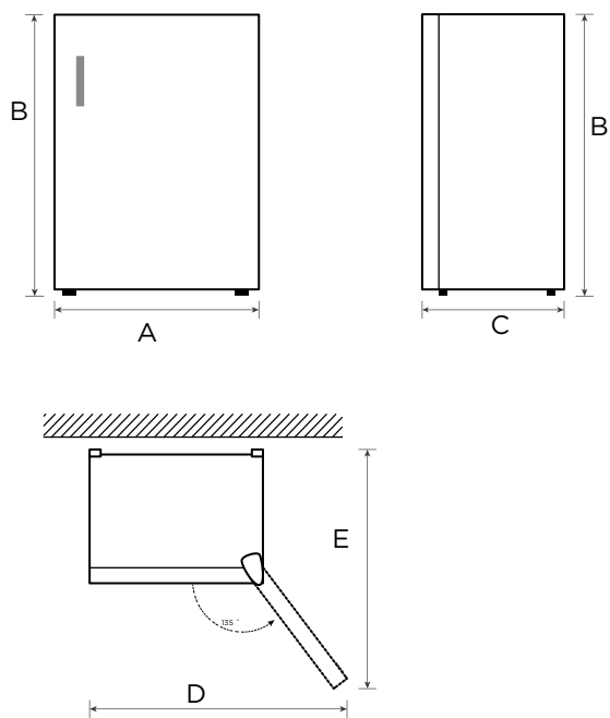
Diagrama do espaço necessário (com a porta aberta e com a porta fechada)
