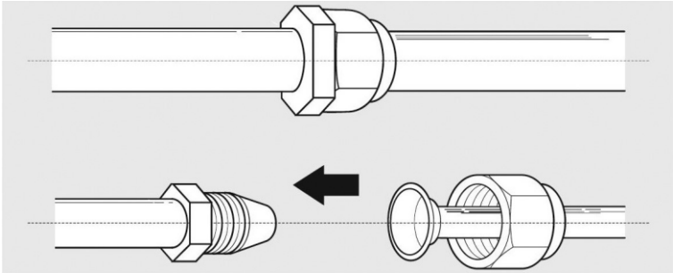
Fig. 4.6 conexión de la tubería que transporta refrigerante
