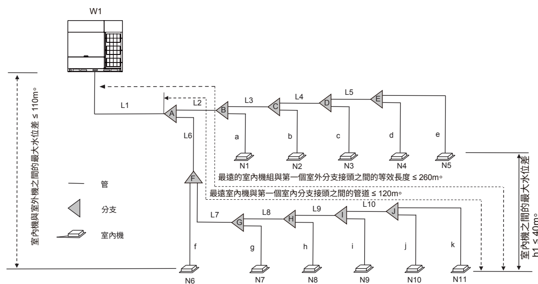
V8i 個別系列的管道圖
