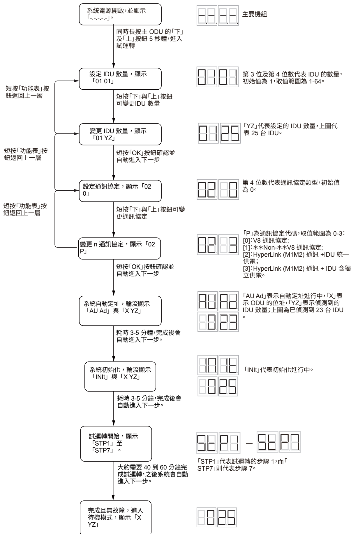
試運轉流程圖
