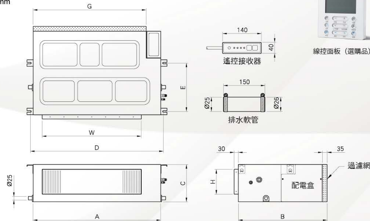
送風機三視尺寸圖
